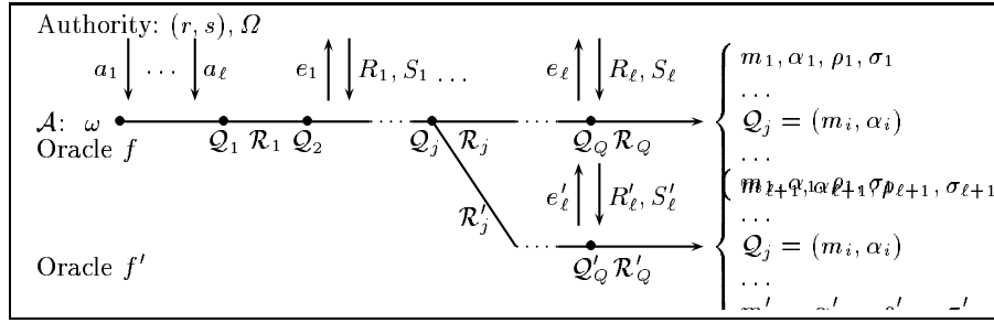
Fig. 12. Forking Lemma.
