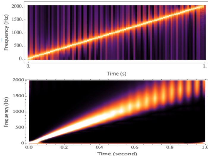
FIGURE 35 – Comparaison entre une analyse par fenêtrage dont la taille de boîte d'inspection est fixe (haut), et une analyse par ondelettes (bas) où la taille de boîte évolue selon le schéma de la figure 34. Le signal x(u) = \sin(2000\pi u^2) échantillonné au rythme de 1/4095 sur u \in [0, 1] . Pour la TO, on a utilisé une ondelette de Gabor 1/\pi^{1/4}e^{-u^2/2}e^{i\xi u} avec \xi = 6 .
