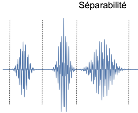
FIGURE 24 – Exemple de l’usage de la séparabilité pour isoler les signaux où il y a de l’information, et sur chaque intervalle on peut procéder à une représentation parcimonieuse (sparcité).
