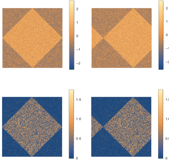
FIGURE 21 – Illustration de la propriété d'équivariance de non-linéarité ponctuelle: (haut) de gauche à droite: image origine, image translatée; (bas) de gauche à droite: rectification (ReLU) de l'image d'origine, et rectification de l'image translatée.
