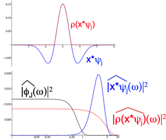
FIGURE 45 – Illustration de l’effet d’un ReLU sur la convolution x * \psi_{aj} . En haut, le résultat dans l’espace réel, et en bas ce qui se passe dans l’espace de Fourier. Avec le ReLU, la composante basse fréquence produit avec le filtre passe-bas \phi_J donne une contribution non nulle (ici pour faire simple on a pris x(u) = \delta(u - u_0) donc la convolution redonne l’ondelette translatée.
