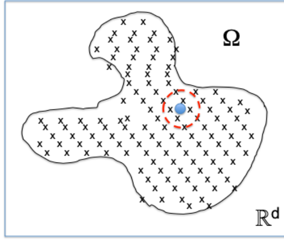
FIGURE 11 – Pavage de l'espace \Omega à l'aide de boule de rayon \varepsilon .
