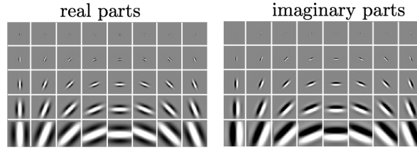
FIGURE 52 – Représentation d'ondelettes complexes dilatées et tournées.
