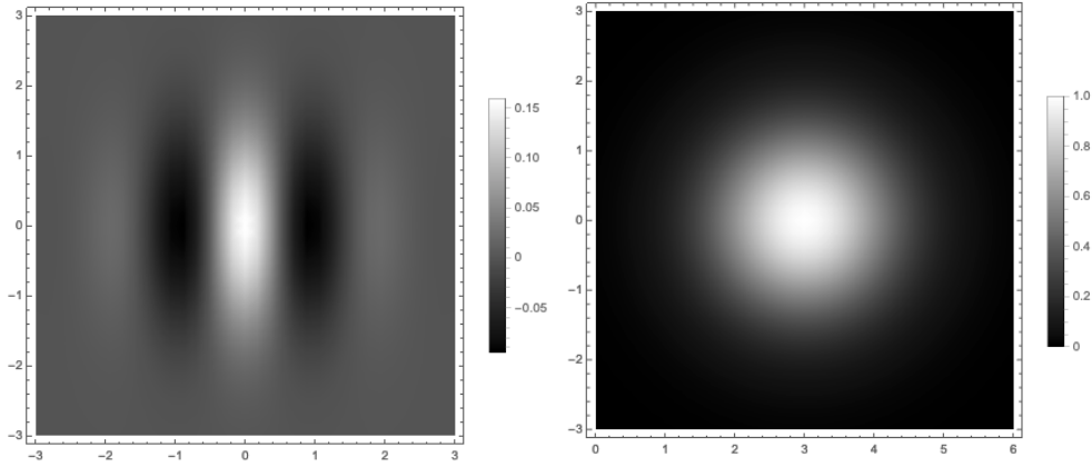
FIGURE 46 – Exemple d'ondelette bidimensionnelle \mathcal{N}_{(0,1)}(x,y)e^{i3x} : à gauche la partie réelle, à droite la transformée de Fourier (notez que l'on obtient un gaussienne décalée selon l'axe horizontal de 3 unités).
