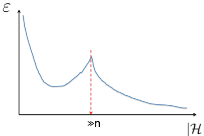
FIGURE 8 – La borne supérieure classique est battue dans les réseaux de neurones très profond, au delà d'une taille critique, l'erreur diminue au lieu de s'envoler.
