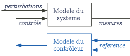
(1) Modélisation
