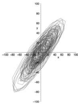
trace d'exécution
