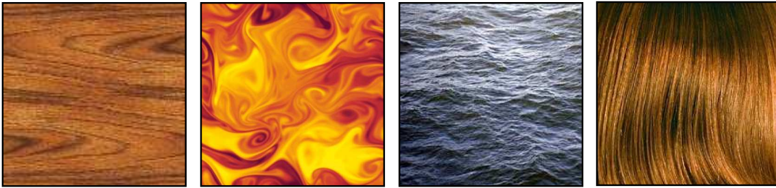
FIG. 21 – Exemples de textures avec des géométries complexes à longue portée.
