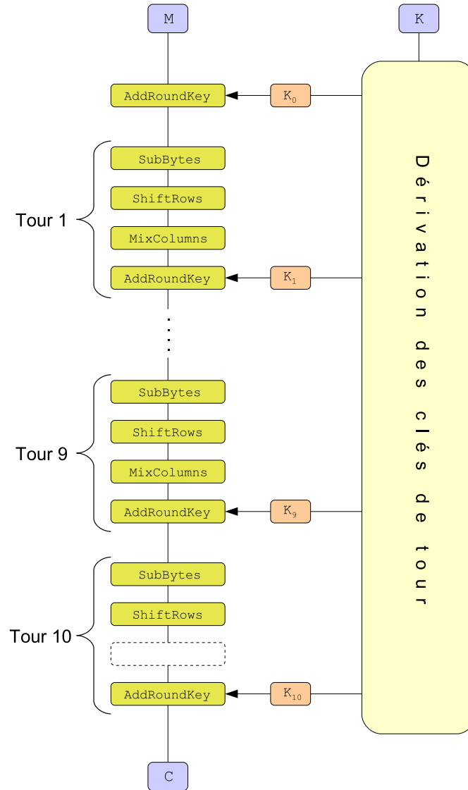
FIG. 1.8 – L’algorithmhe AES.
