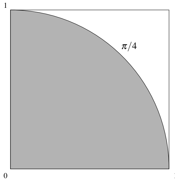
Figure 5.1: Calcul de \pi/4 par la méthode de Monte-Carlo.
